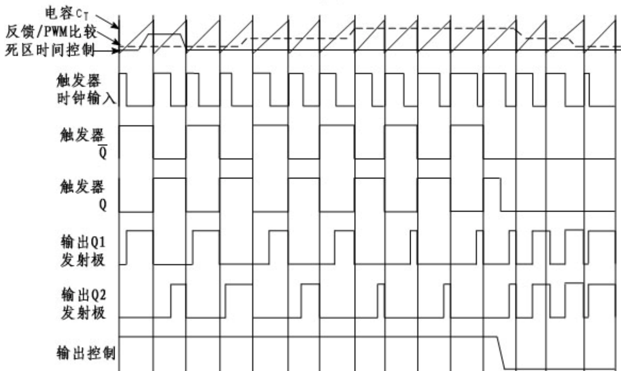
图2. 时序图
