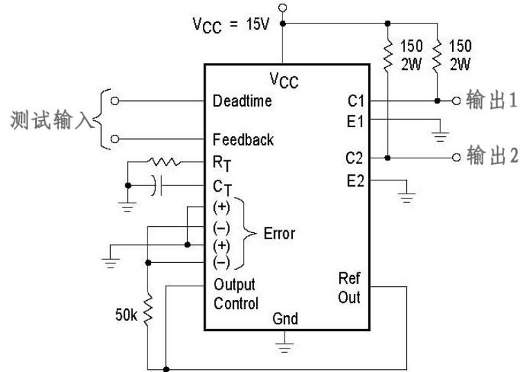
图11. 死区时间和反馈控制电路
