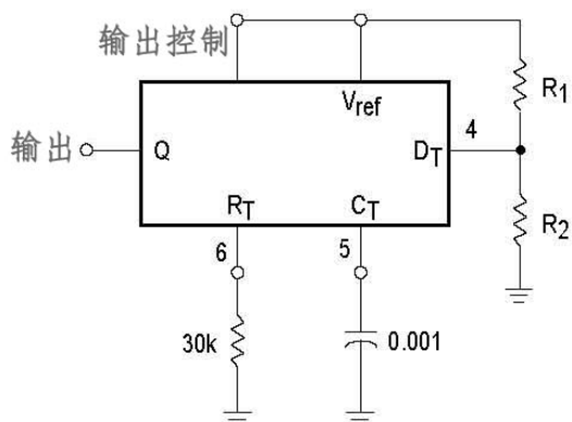
图15. 死区时间控制电路
