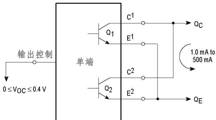
图17. 单端式和推挽式的输出连接方法
