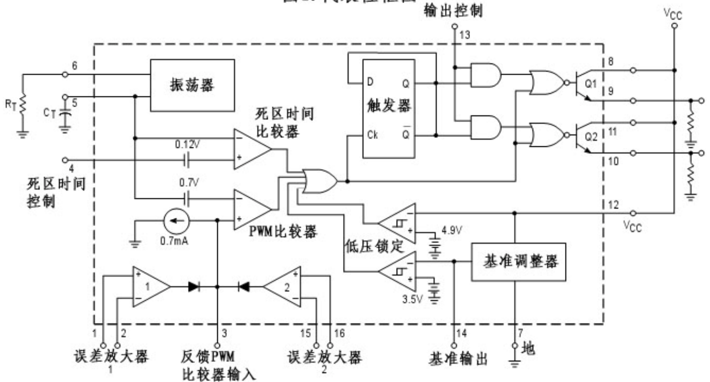
图1. 代表性框图
